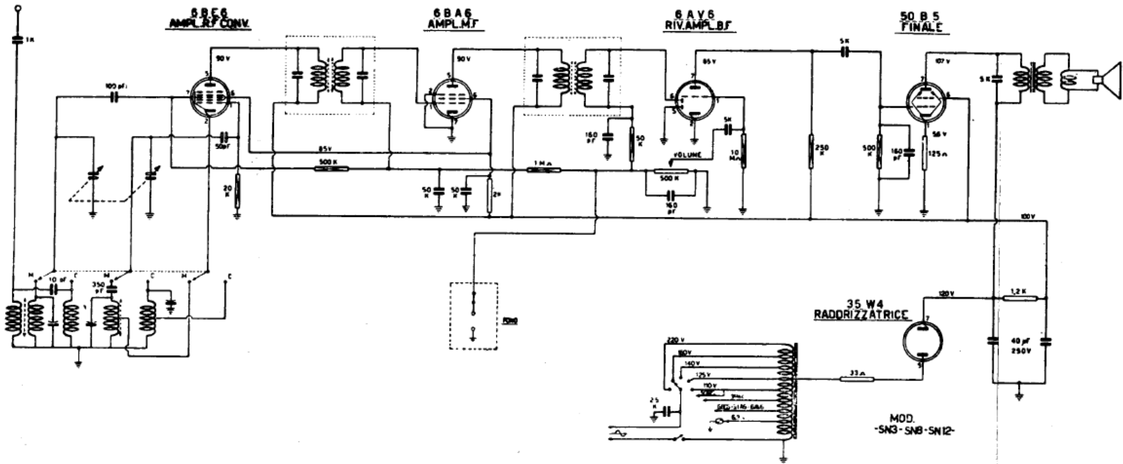
ULTRAVOX - Modd. SN 3, SN 8 e SN 12. Apparecchi a modulazione di ampiezza, con una gamma onde medie e una banda onde corte. Media frequenza a 468 kc/s. Resa d'uscita 2 watt. Consumo 45 watt.
